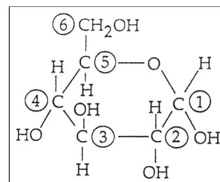
Fig. 3. Cellulose unit.
